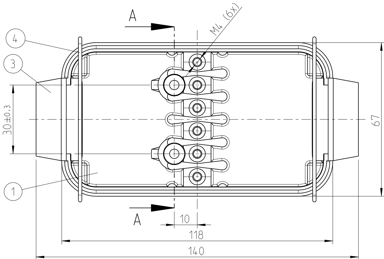
Ansicht ohne Deckel VIEW WITHOUT COVERS
